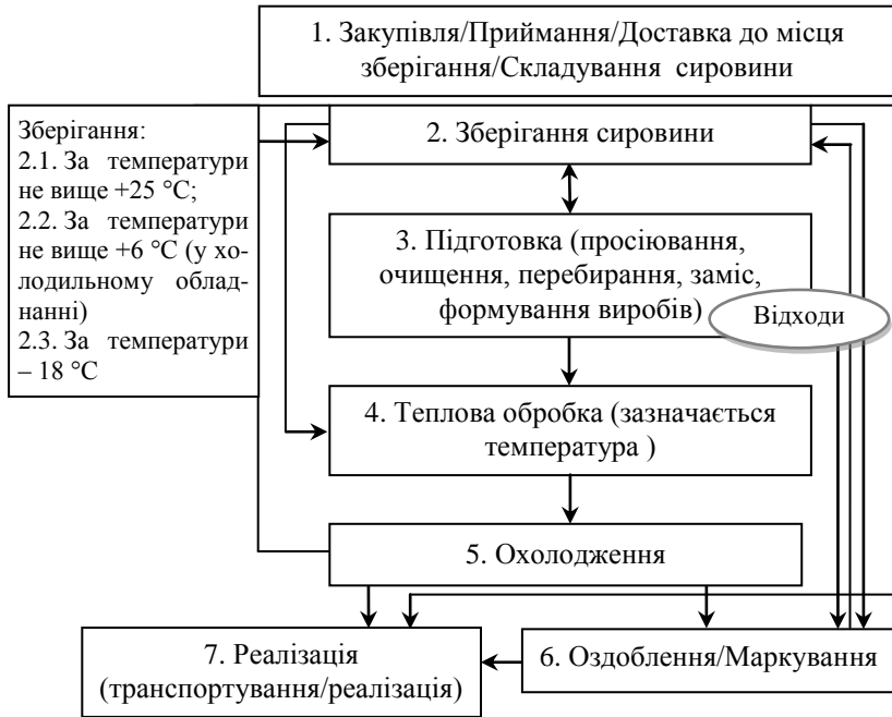
Рисунок 19 – Приклад блок-схеми технологічного процесу виробництва
